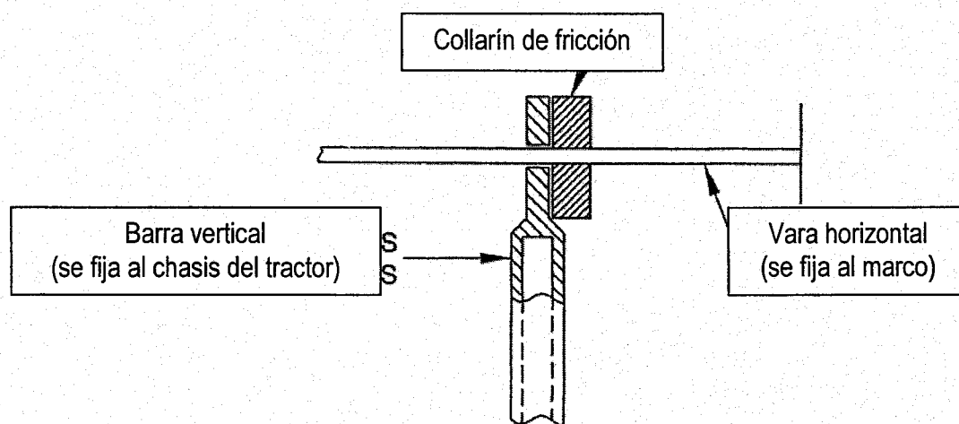
Figura C-4 Método para medir la deflexión instantánea
