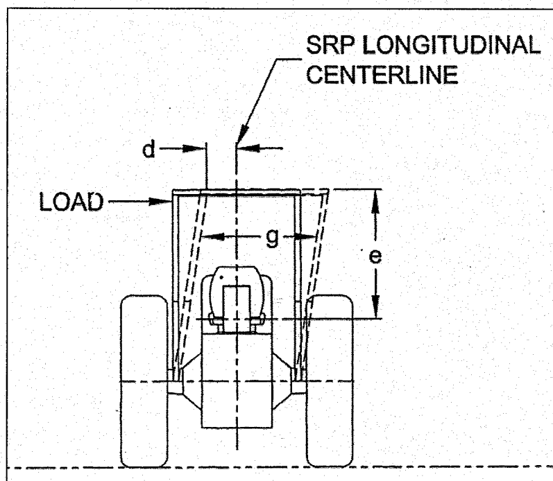
Figura C-2 Aplicación de carga lateral
