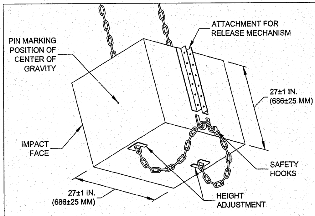
Figura C-6: Péndulo
