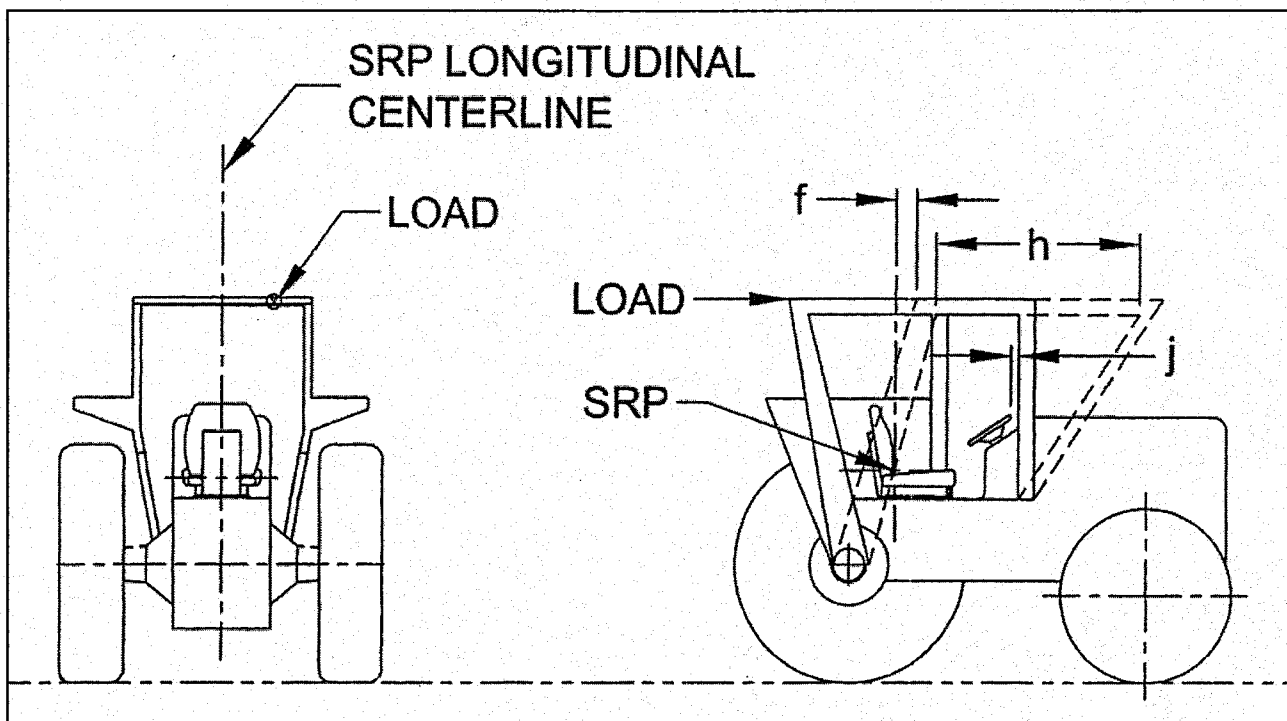
Figura C-14 Aplicación de carga posterior
