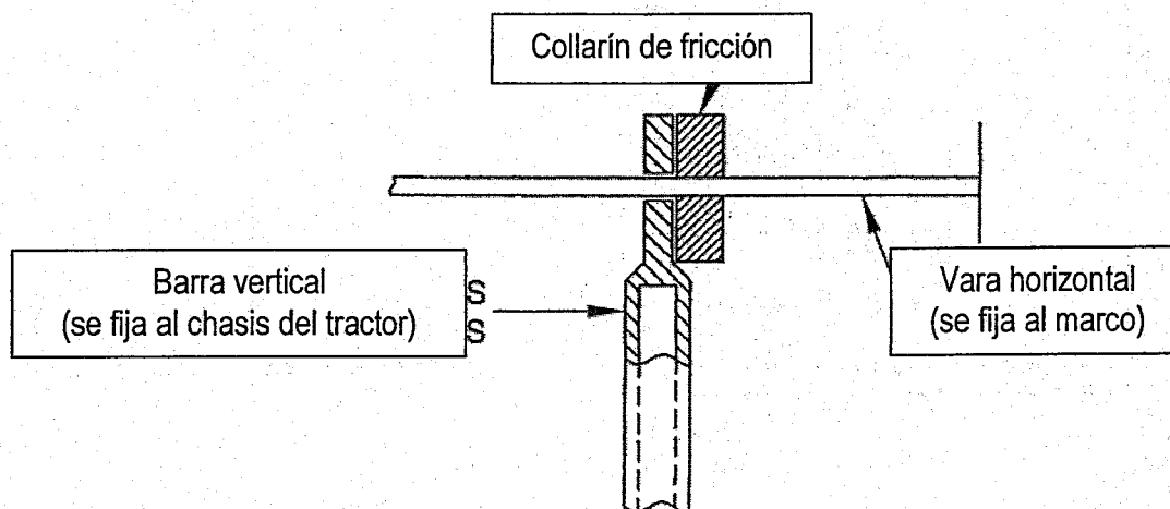
Figura C-4 Método para medir la deflexión instantánea
