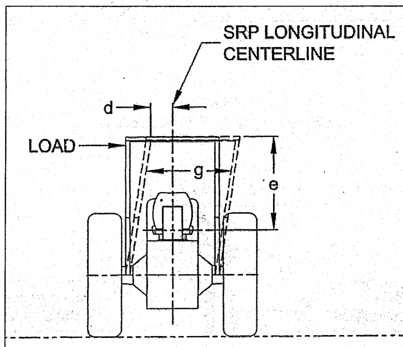
Figura C-2 Aplicación de carga lateral
