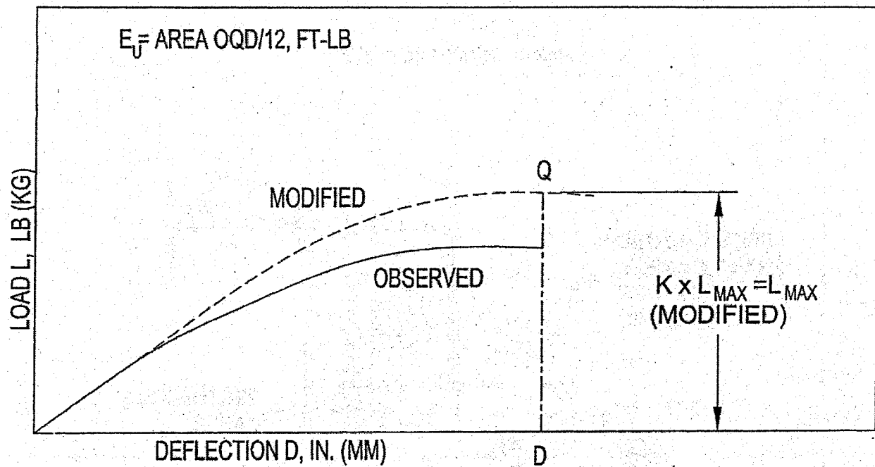
Figura W-20 Diagrama L_M - D_M característico
