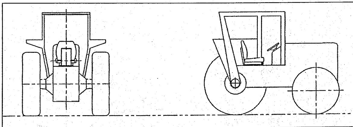
Figura C-12 Tractor con recinto protector característico
