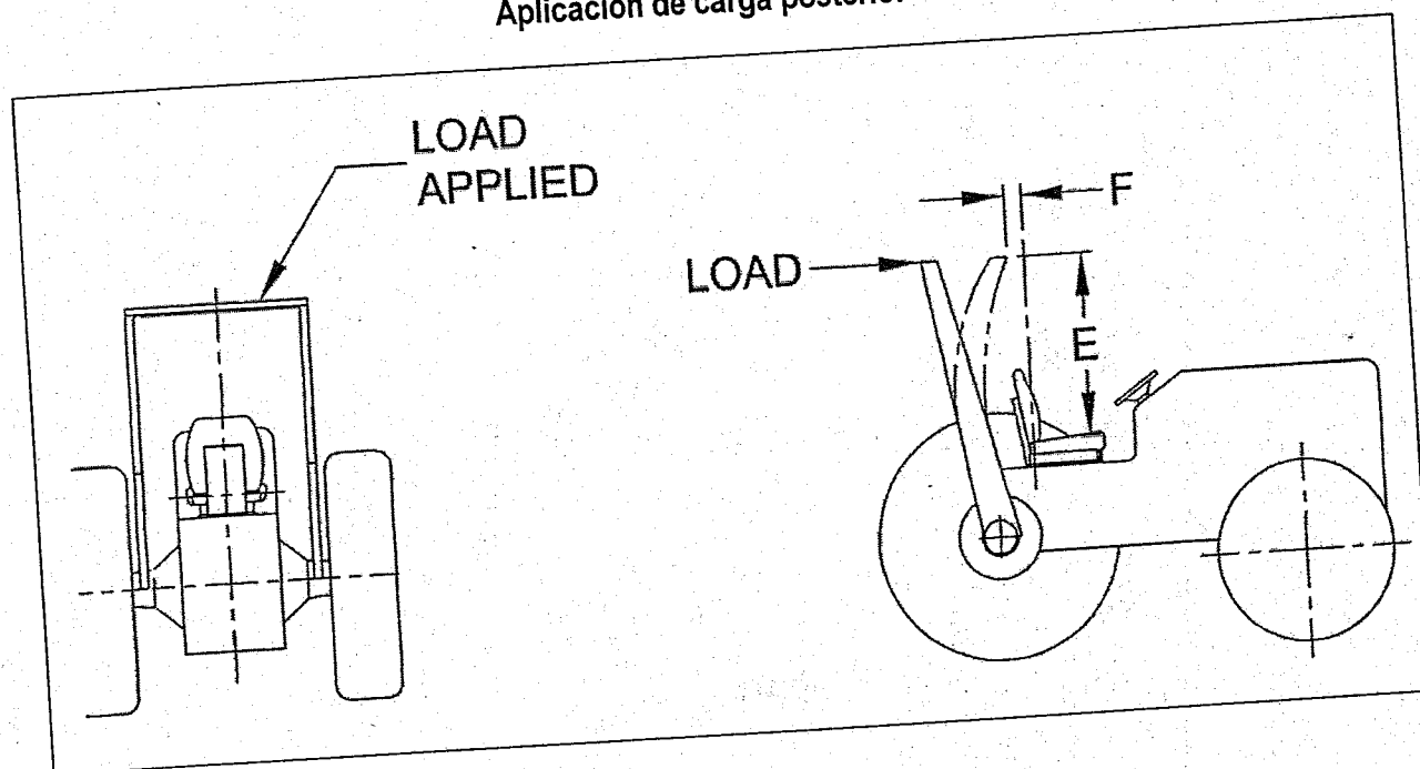
Figura W-18: Método para medir la deflexión instantánea
