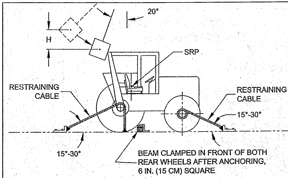
Figura C-15 Aplicación de impacto posterior
