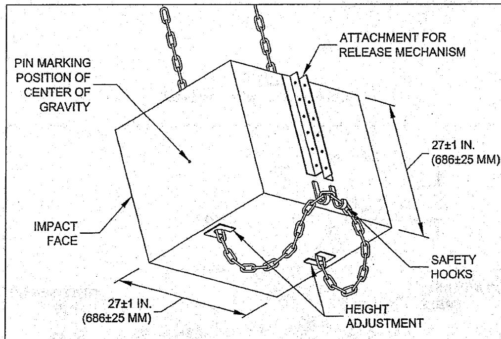
Figura C-6: Péndulo
