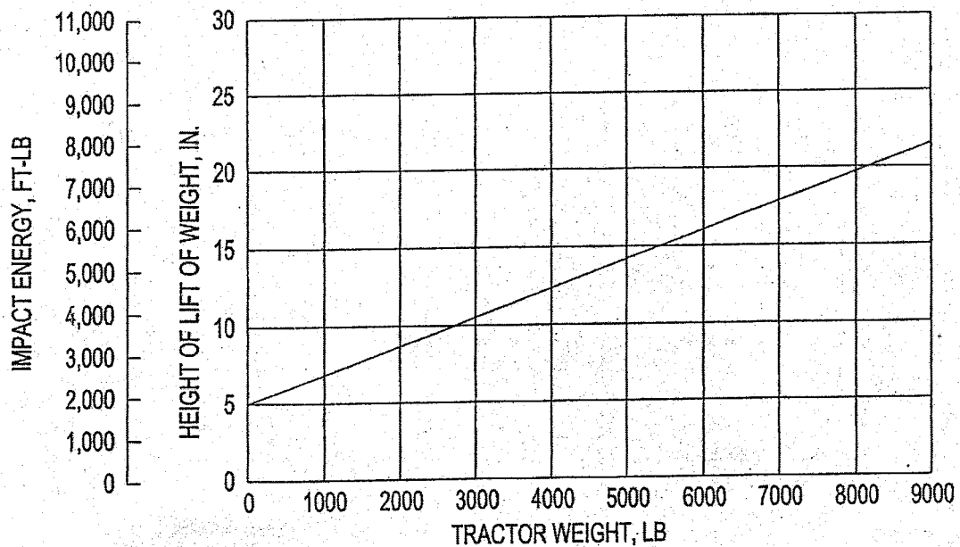
Figura W-24 Energía de impacto y altura de levantado correspondiente de una pesa de 4,410 lb (2,000)
