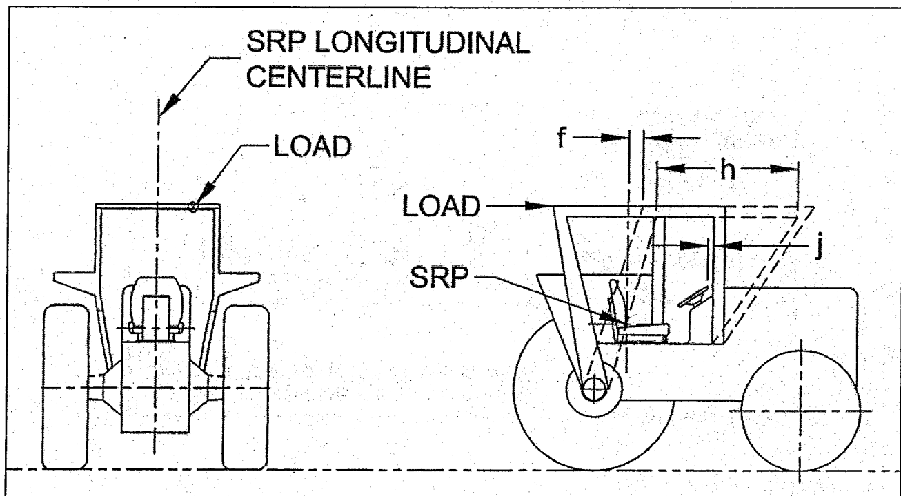
Figura C-14 Aplicación de carga posterior
