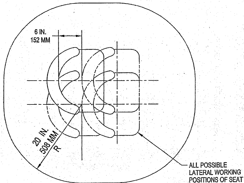
Figura W-26 Zona de protección de la prueba de caída.
