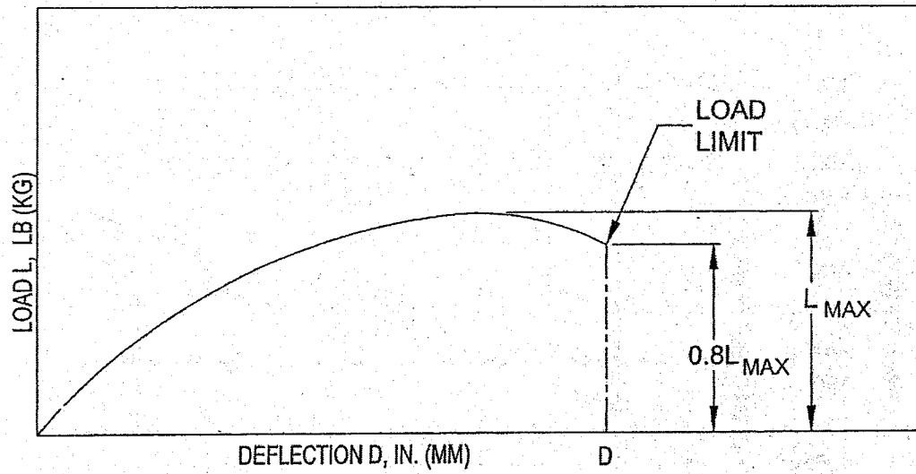
Figura C-5 Diagrama característico L-D
