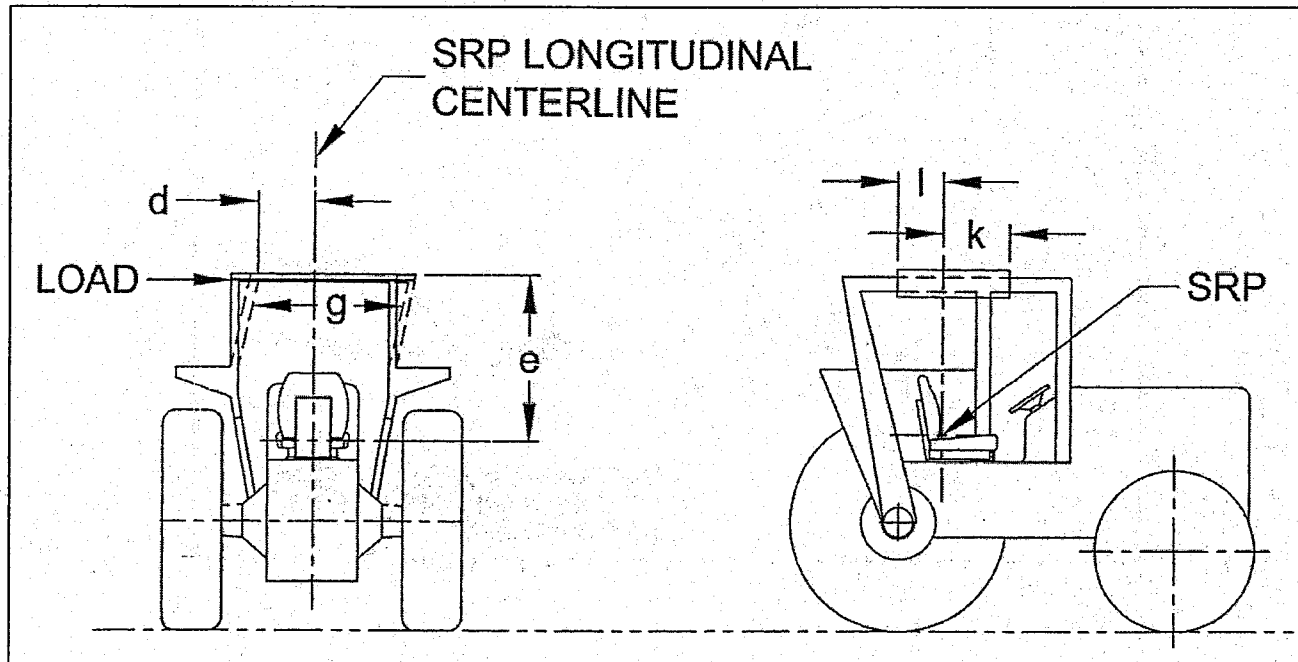
Figura C-13 Aplicación de carga lateral
