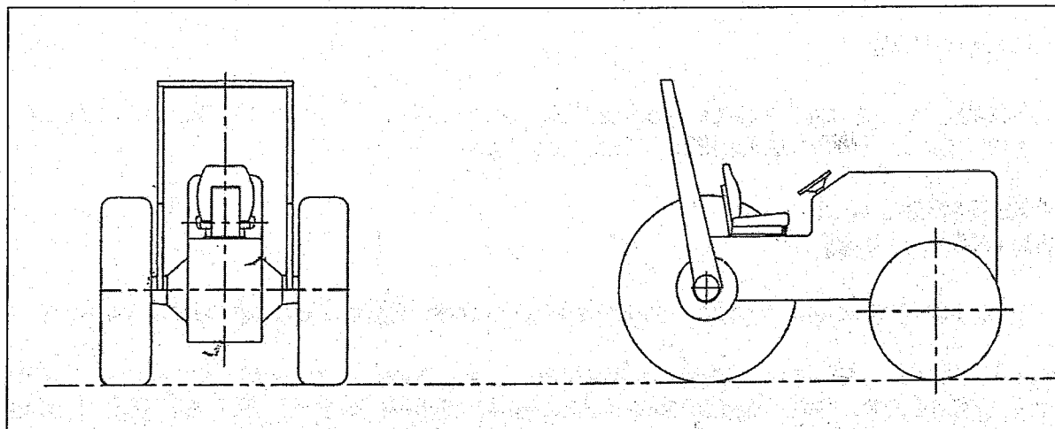
Figura W-14 Configuración característica del marco
