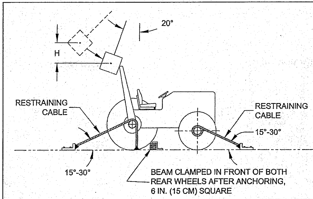
Figura W-23 Método de impacto lateral
