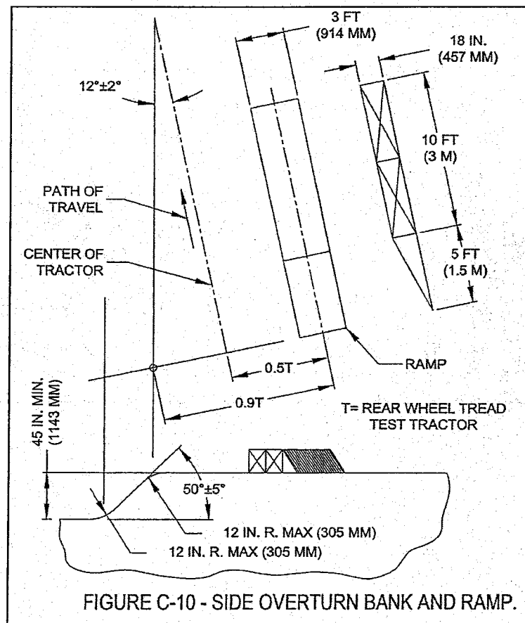
Figura C-10 Banco y rampa de vuelco lateral
