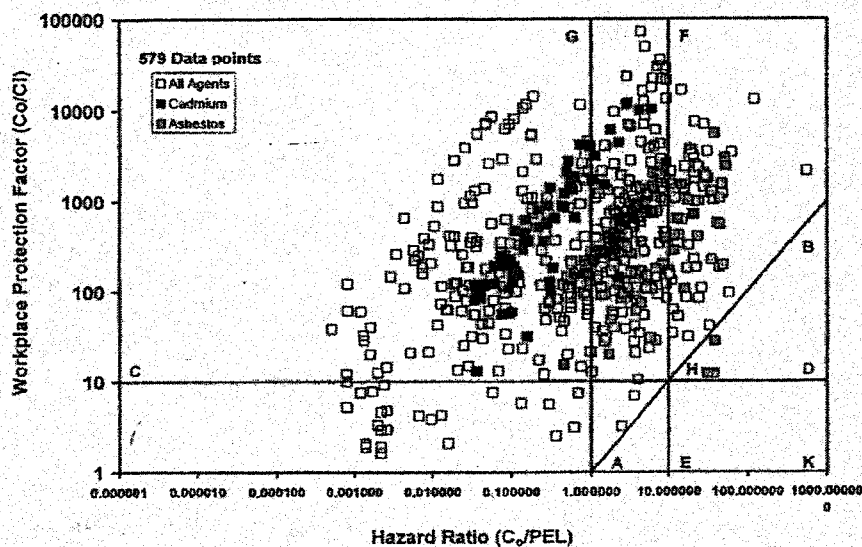
Figura 5. Respiradores elastoméricos (PELs antes de abril de 1993)
