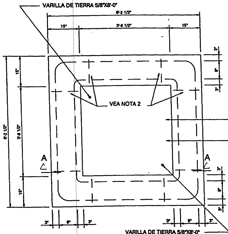
PLANTA
