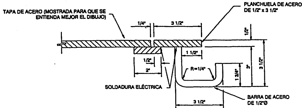
DETALLE 1
