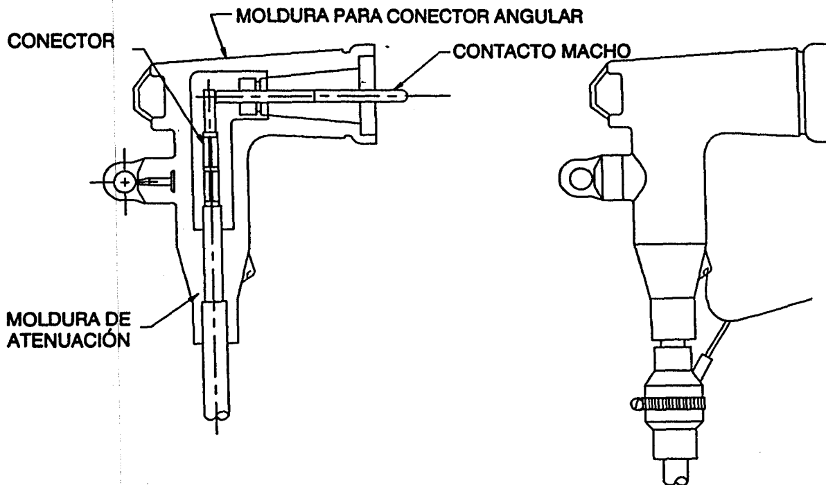
VISTA EXTERNA
