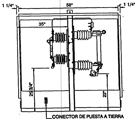
SECCIÓN "A"
