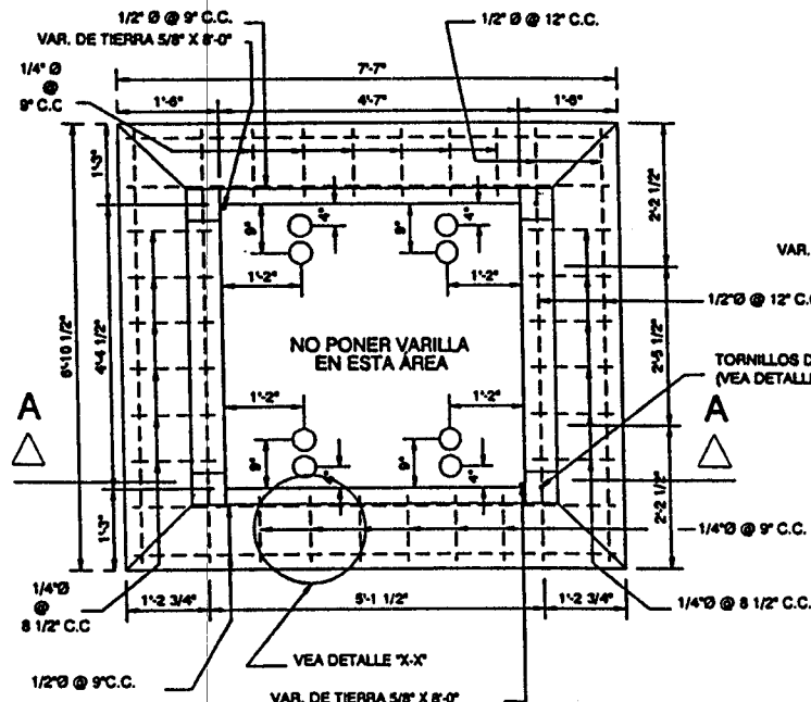
VISTA DE TOPE
