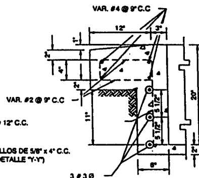
DETALLES "X-X" NO A ESCALA
