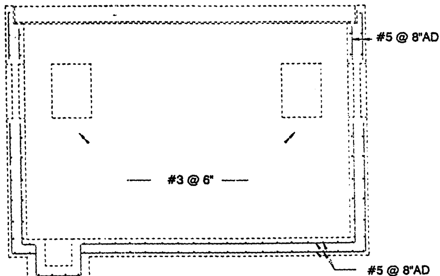
SECCIÓN "A-A"
