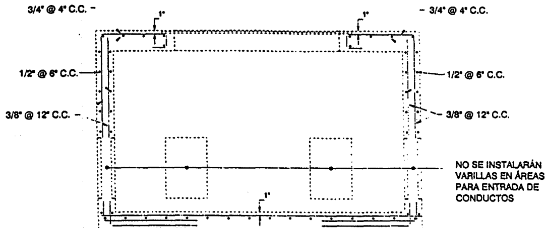
SECCIÓN "A-A"
