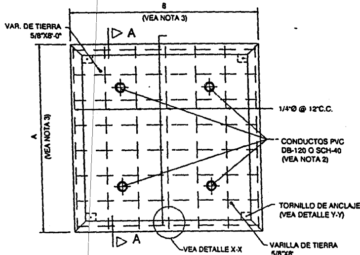
PLANTA NO A ESCALA
