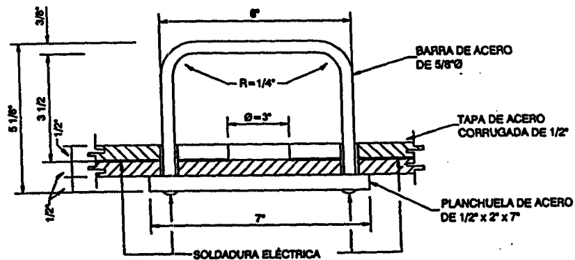
DETALLE 2 ELEVACIÓN
