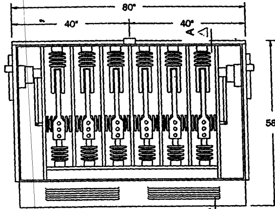
VISTA FRONTAL (PUERTAS REMOVIDAS)
