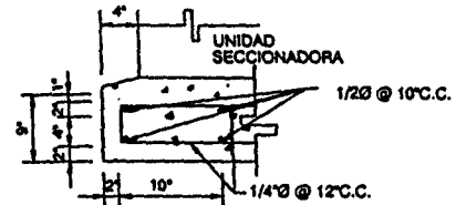
DETALLE "X-X" NO A ESCALA
