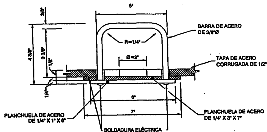
ELEVACIÓN
