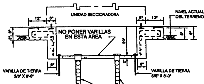
SECCIÓN "A-A" NO A ESCALA
