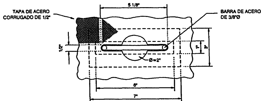
PLANTA
