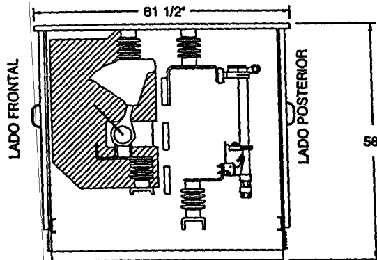
SECCIÓN "A"
