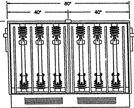
VISTA POSTERIOR (PUERTAS REMOVIDAS)
