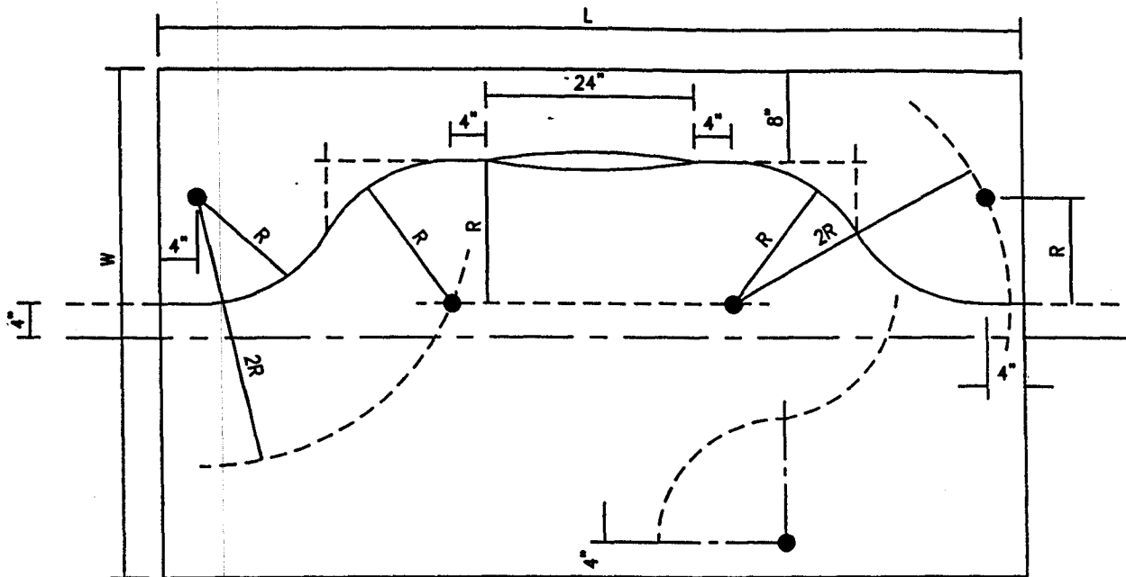
PROCEDIMIENTO GRÁFICO PARA DETERMINAR LAS DIMENSIONES DEL REGISTRO EN FUNCIÓN DEL DIÁMETRO EXTERIOR DE LOS CABLES
