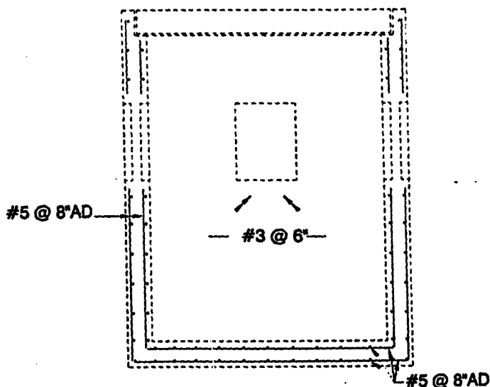
SECCIÓN "B-B"
