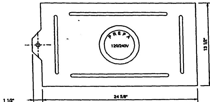
VISTA SUPERIOR
