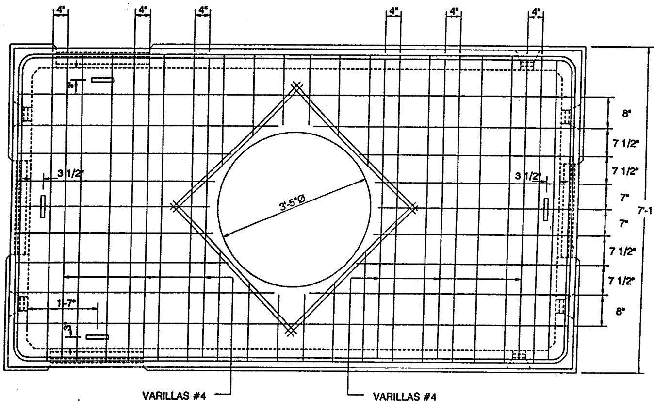
VISTA SUPERIOR
