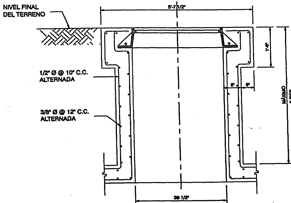
SECCIÓN "A-A"
