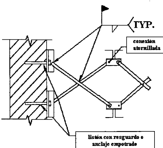
conexión en puente diagonal atornillada en una pared
