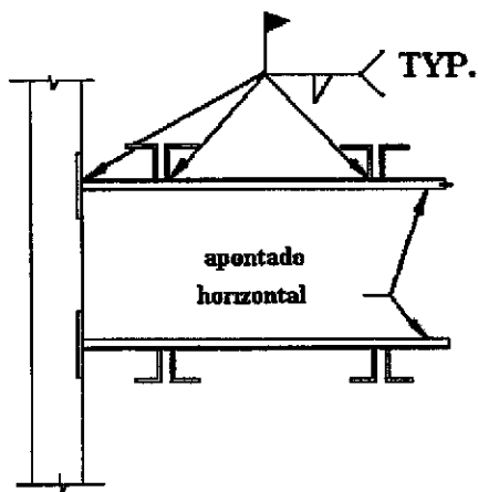
conexión en puente horizontal en una pared de paneles
