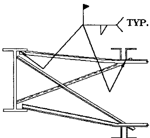
conexión en puente horizontal en una estructura con "apontado en cruceta"
