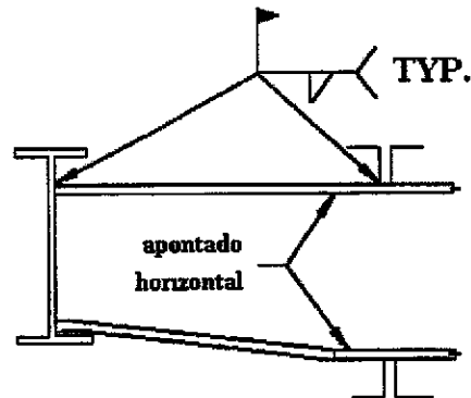
conexión en puente horizontal en una pared
