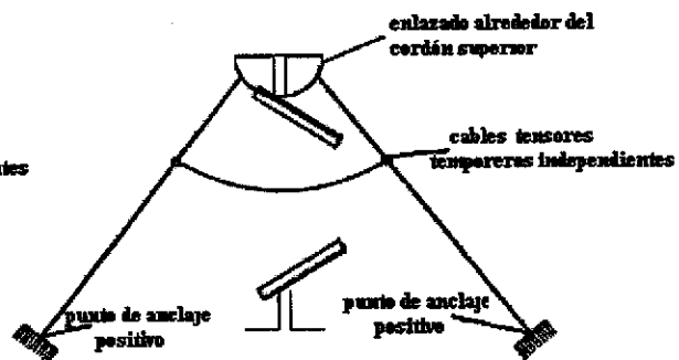
Conexión en puente diagonal asegurada con cables tensores temporeros
