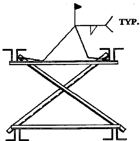
conexión en puente entre dos viguetas
