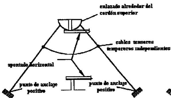
Conexión en puente horizontal asegurada con cables tensores temporeros
