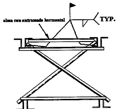
conexión en puente entre dos viguetas con entramado horizontal
