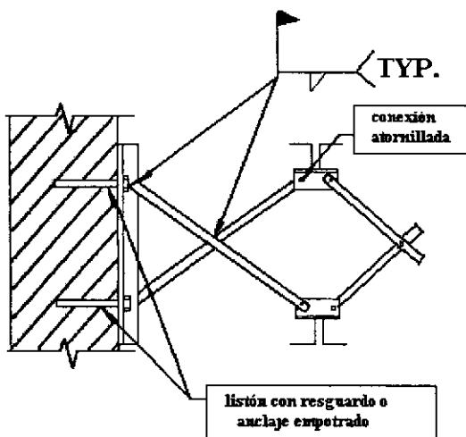
conexión en puente diagonal atornillada en una pared
