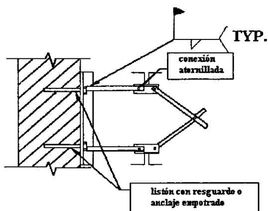
conexión en puente diagonal atornillada en una pared
