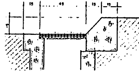
Detalle del Contén en Desagüe Pluvial
