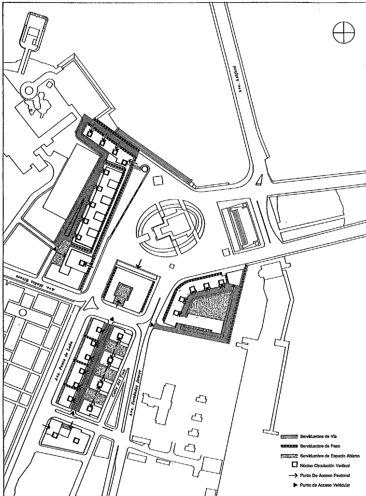
6.0 PLANO DE SERVIDUMBRES Y PUNTOS DE ACCESO
