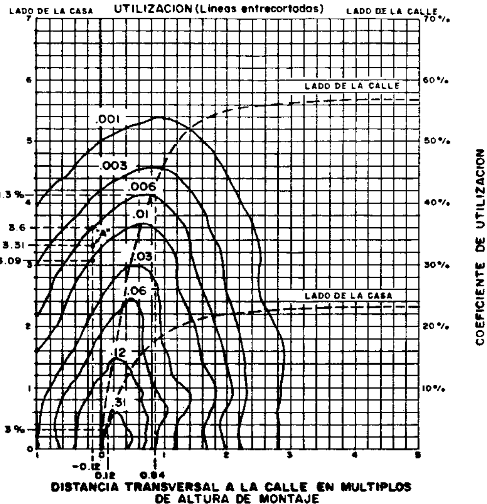
CURVAS DE ISO-PIE-BUJIAS Y DE UTILIZACION DISTANCIA DE PRUEBA-25 PIES (7.62 m)
