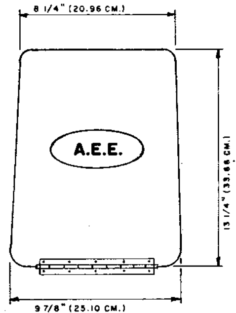
PUERTA VISTA FRONTAL
