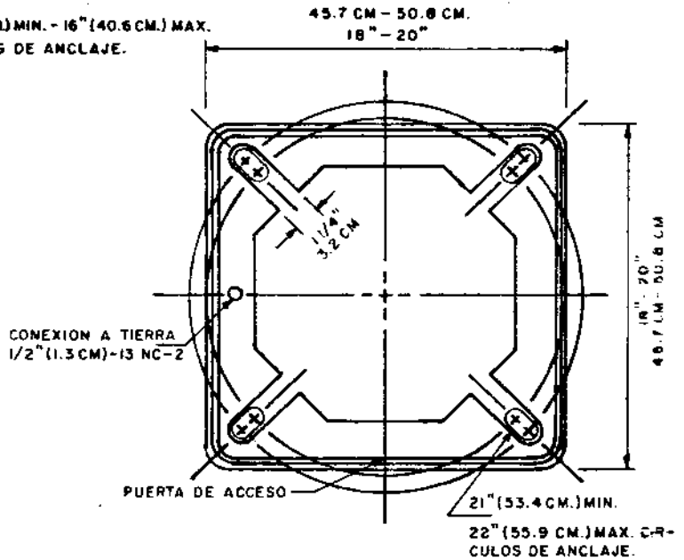
SECCION A - A
