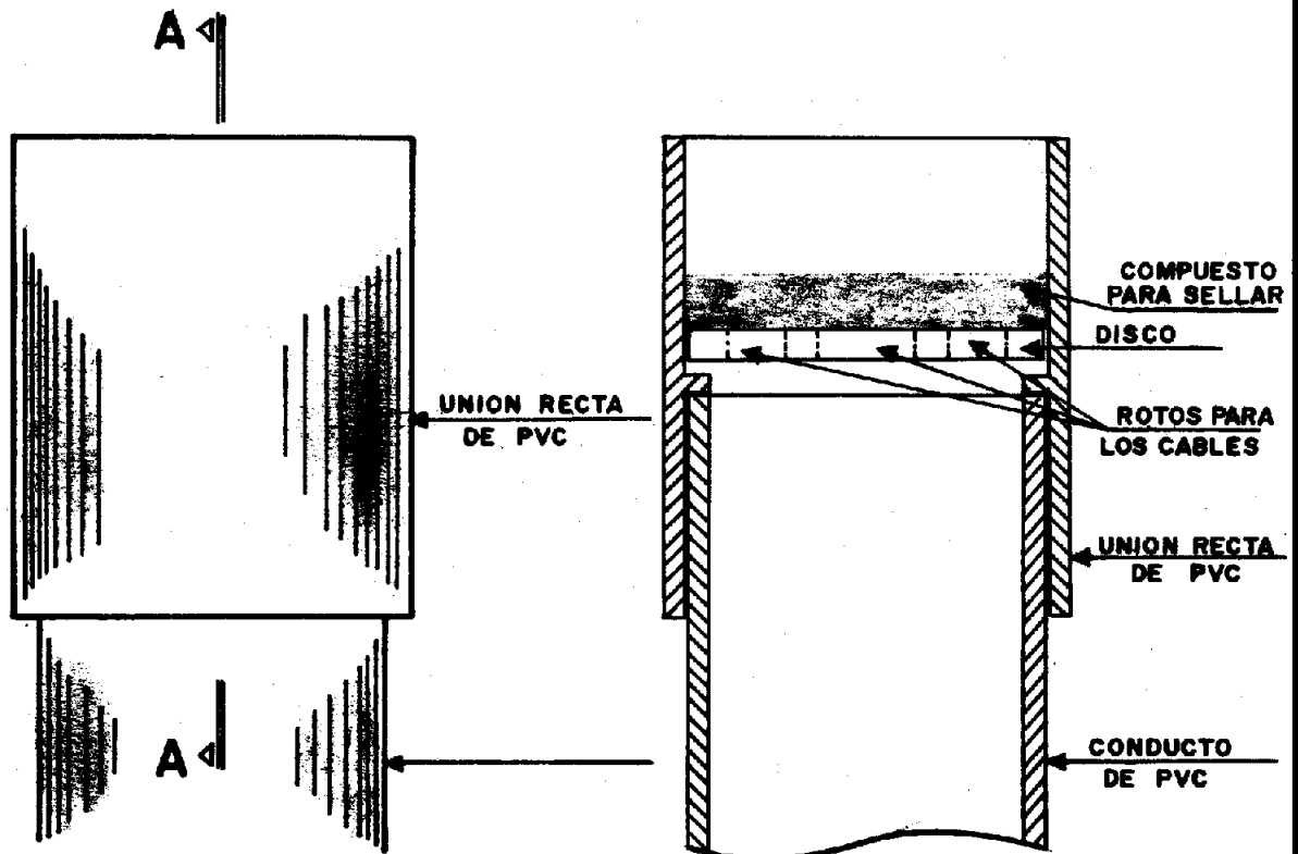
DETALLE DEL SELLO
