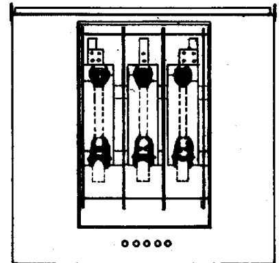
VISTA POSTERIOR (LAS PUERTAS REMOVIDAS)
