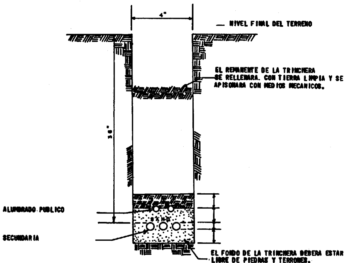
DETALLE DE LA TRINCHERA Y POSICION DE CONDUCTORES
