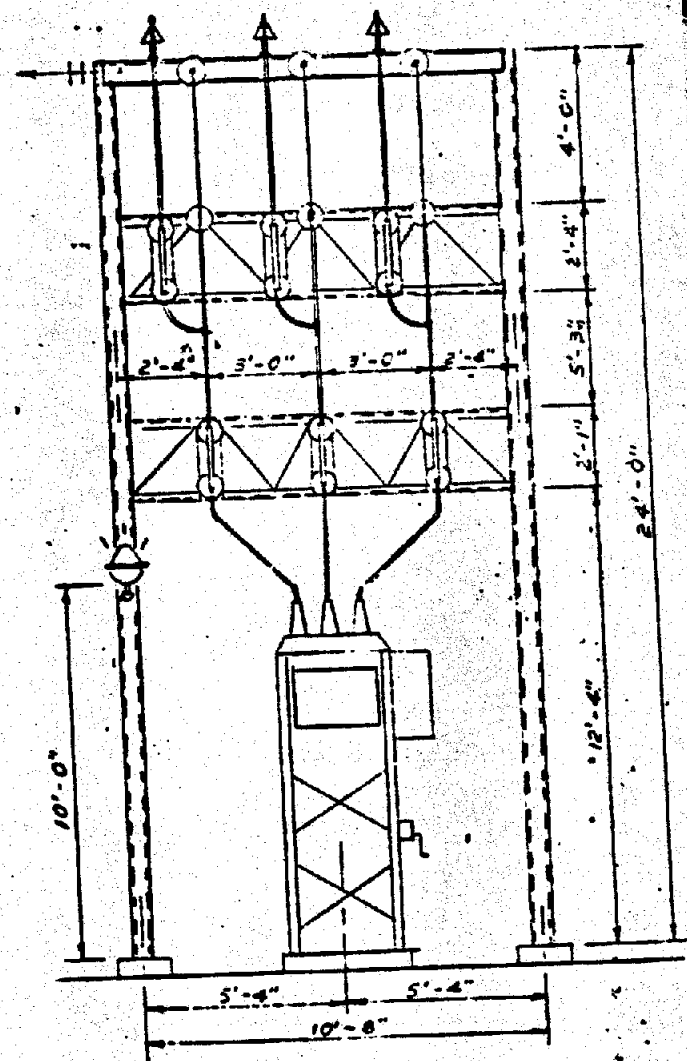
ELEVATION B-B
