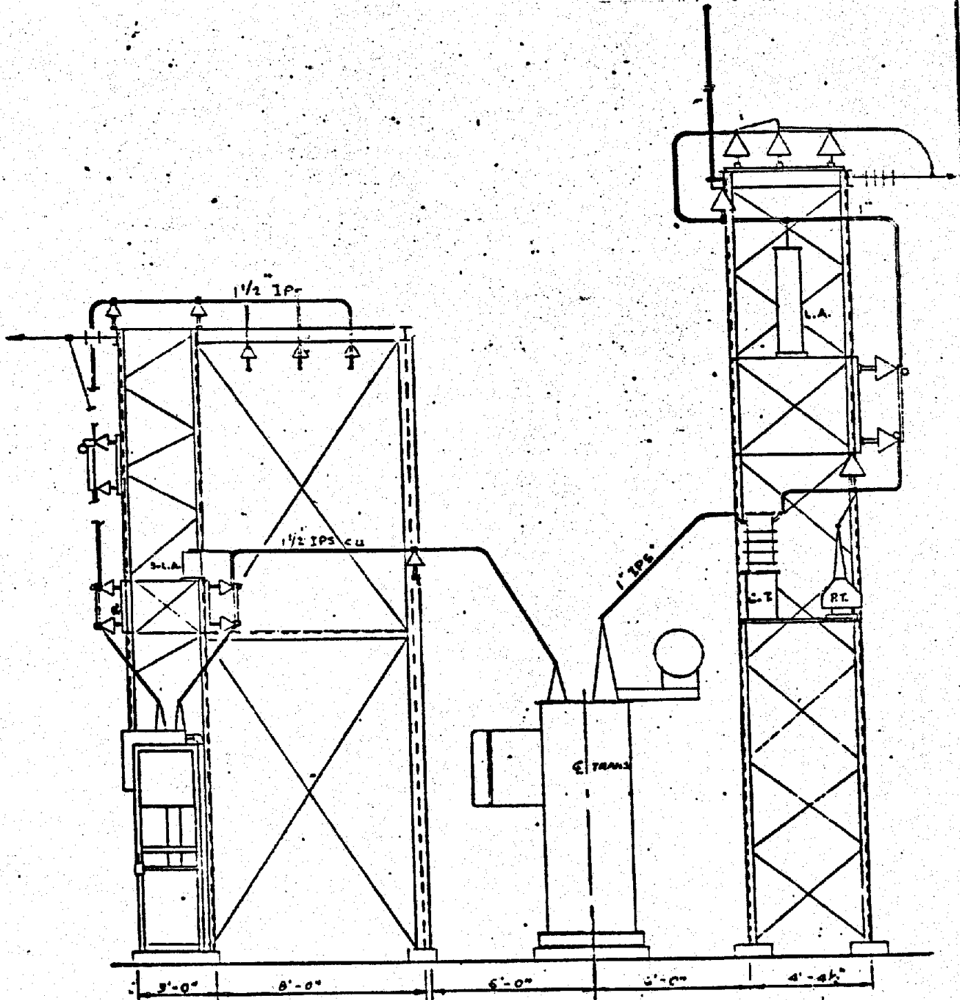
SECTION A-A
