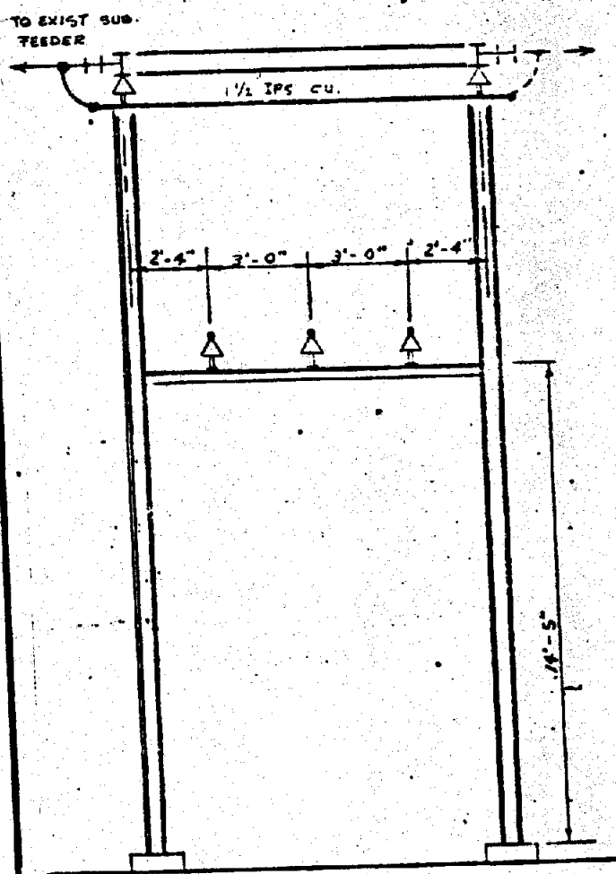
SECTION D-D
