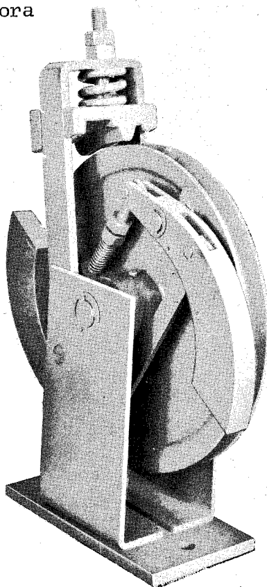
Fig. 2-B:- Regulador Eléctrico de Polea Rotadora.
